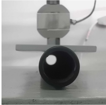
Detalhe: Corpo de prova durante ensaio
