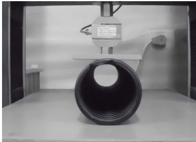
Detalhe: Corpo de prova durante ensaio
